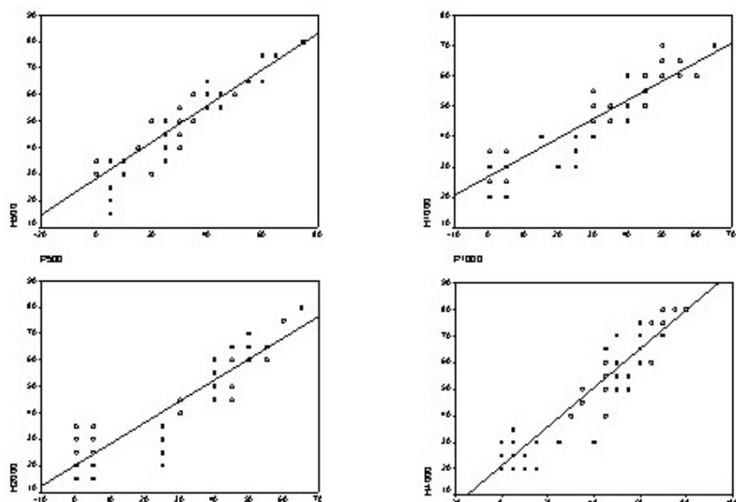
نمودار ۱- منحنی پراکندگی ASSR با ۸۰ هرتز در فرکانس‌های ۵۰۰ تا ۴۰۰۰ هرتز
